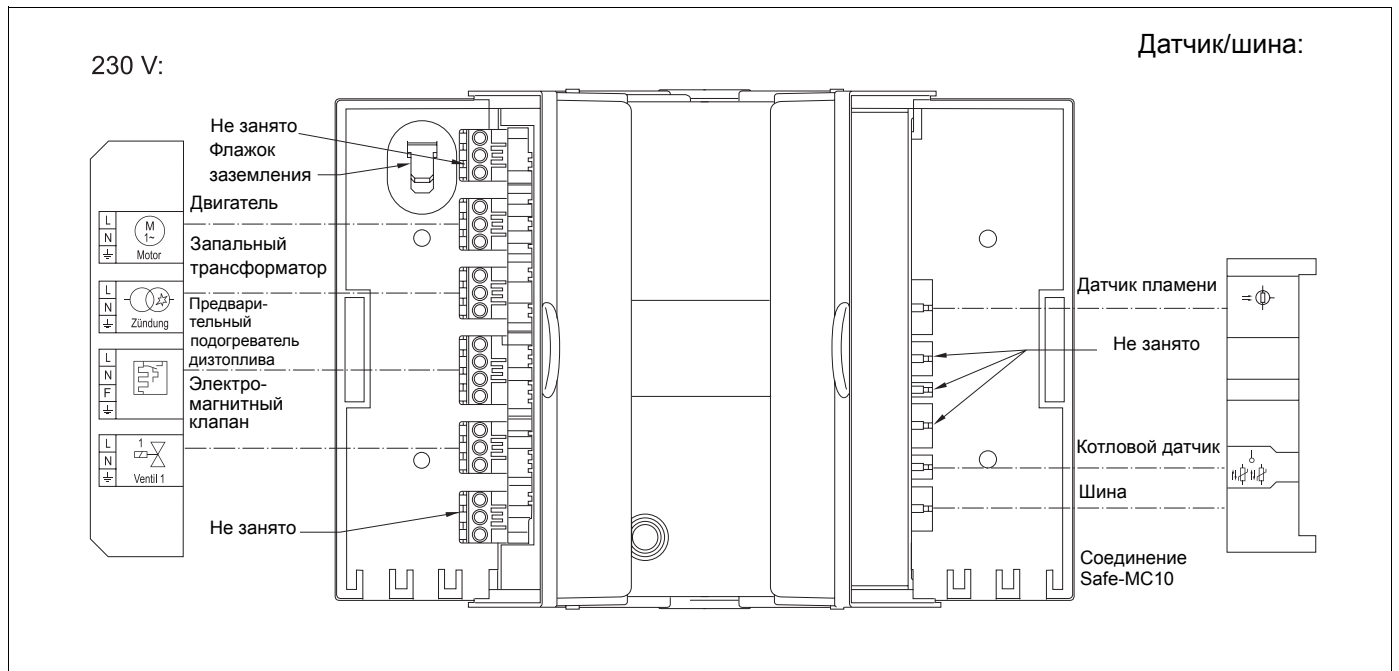
Рис. 11 Схема соединений SAFe 10
