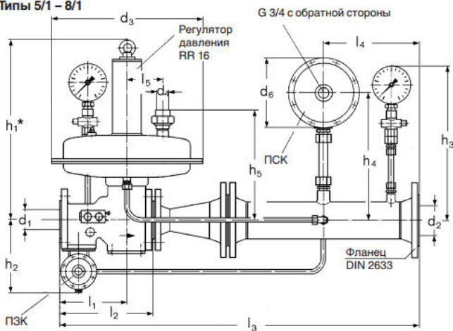
Схема 3 Типы 5/1 – 8/1
