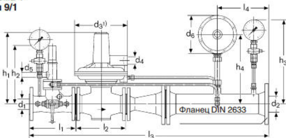
Схема 4 Тип 9/1
